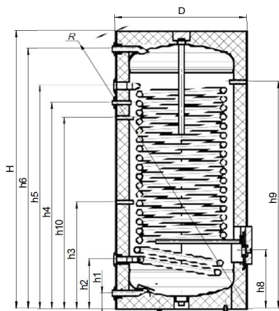
Schéma 1 - Ohříváč vody Triven BTM
