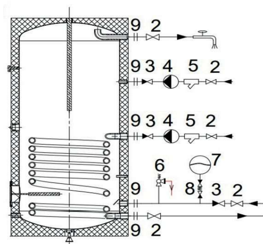
Obrázek 6. Typické doporučené schéma připojení ohřivače vody
